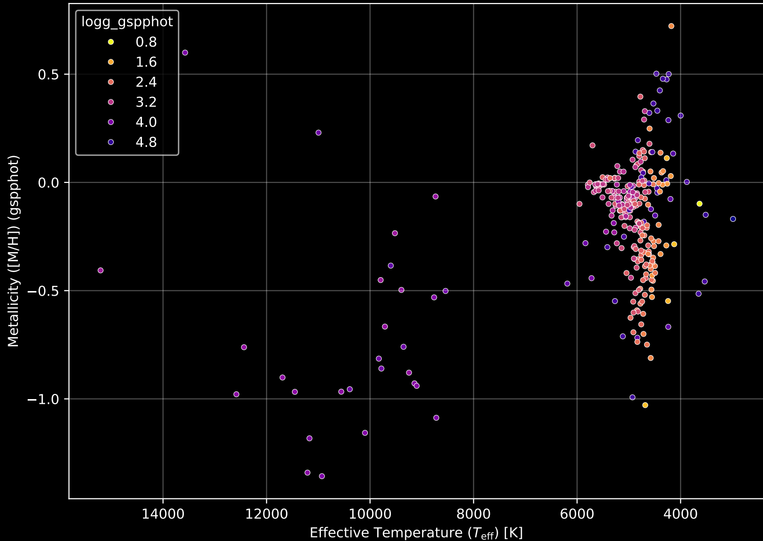
APOGEE DR17 Field: [198+08] Stellar Population Parameters (n= 316)
